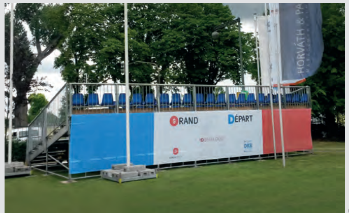
Die mobile Stehtribüne 5 S bei der Tour de France
