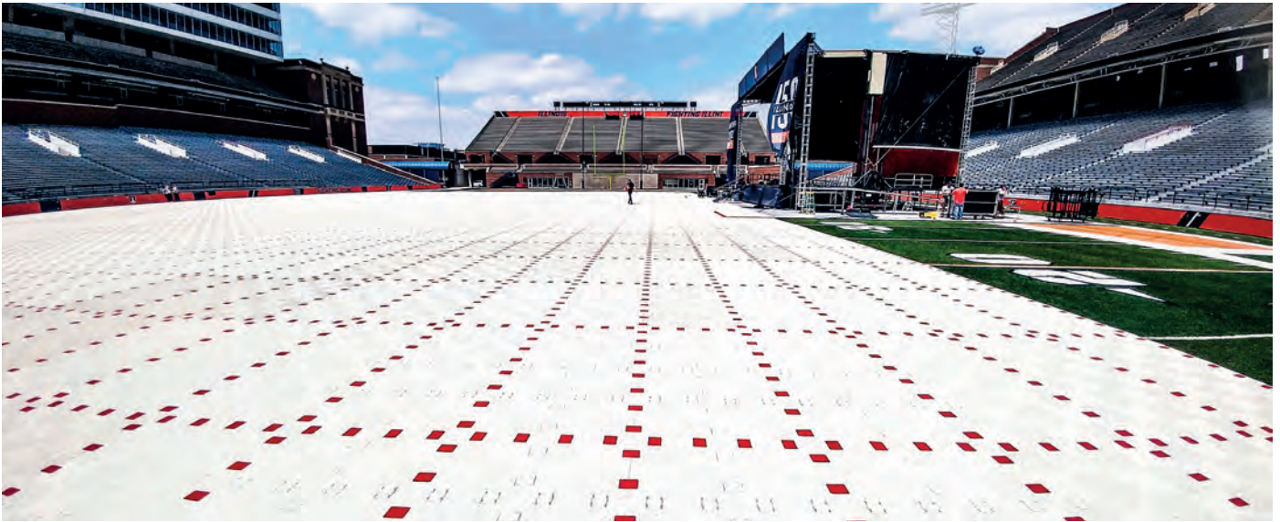
eps Pro im Einsatz als Premiumrasenschutzsystem für ein Open Air Konzert
